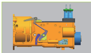
Operação do booster da embreagem hidráulica
